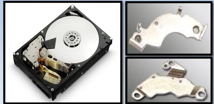
均熱片零件
