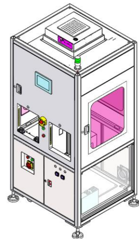
自動貼膜機
